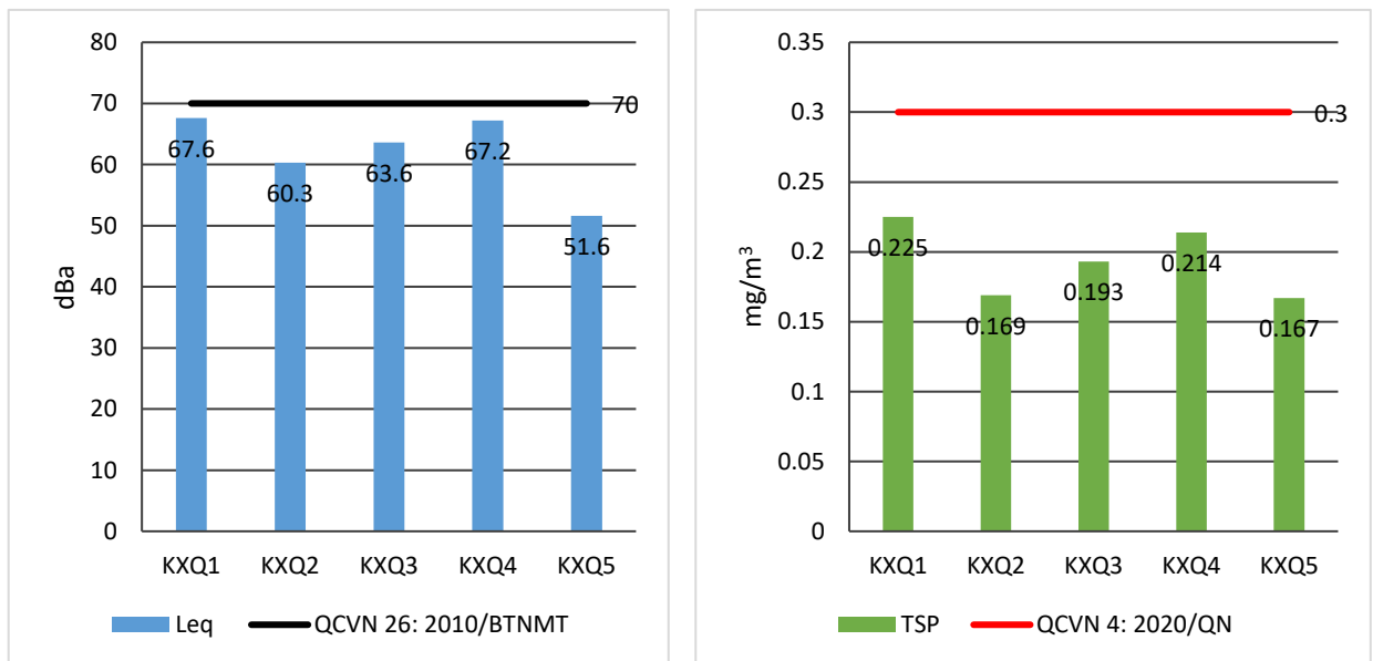
Hình 2.1: Biểu đồ so sánh độ ồn trung bình và hàm lượng bụi lơ lửng với các quy chuẩn tương ứng
