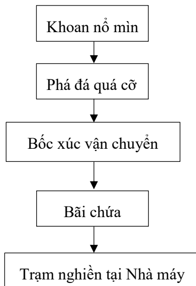
Hình 1.2: Sơ đồ công nghệ khai thác
